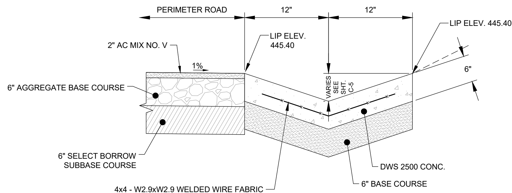
CONC. SWALE DETAIL SCALE: N.T.S.
